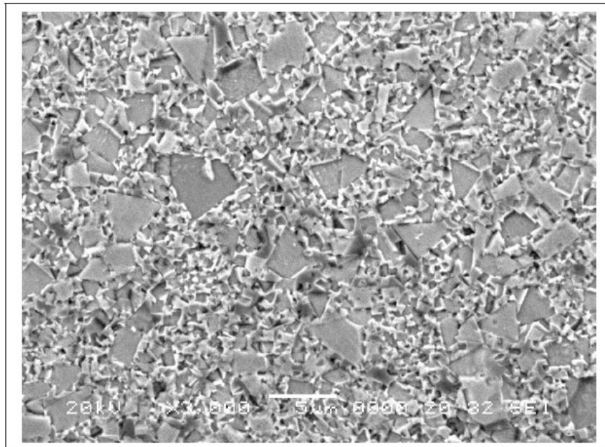
Microstruttura (3000 x)
