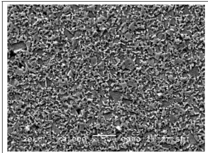
Microstruttura (3000 x)
